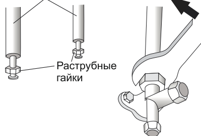
Соединительные трубы
