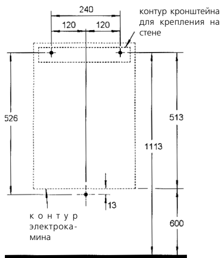
Иллюстрация 2: Рекомендуемые крепежные размеры
