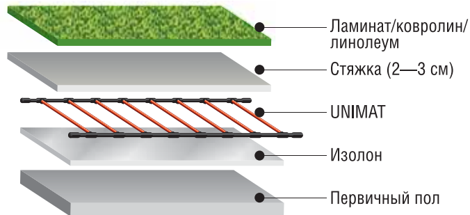
Рис. 21. Схема монтажа теплого пола UNIMAT под ламинат/ ковролин/ линолеум
