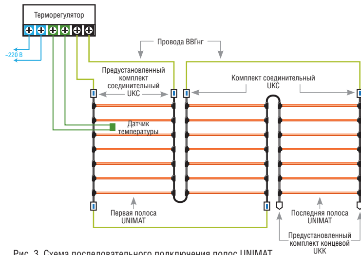
Рис. 3. Схема последовательного подключения полос UNIMAT
