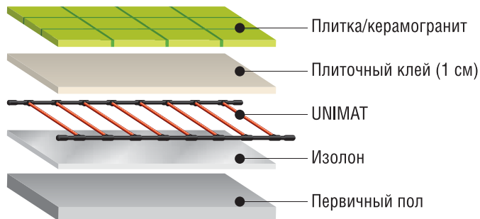
Рис. 23. Схема монтажа теплого пола UNIMAT под плитку/ керамогранит
