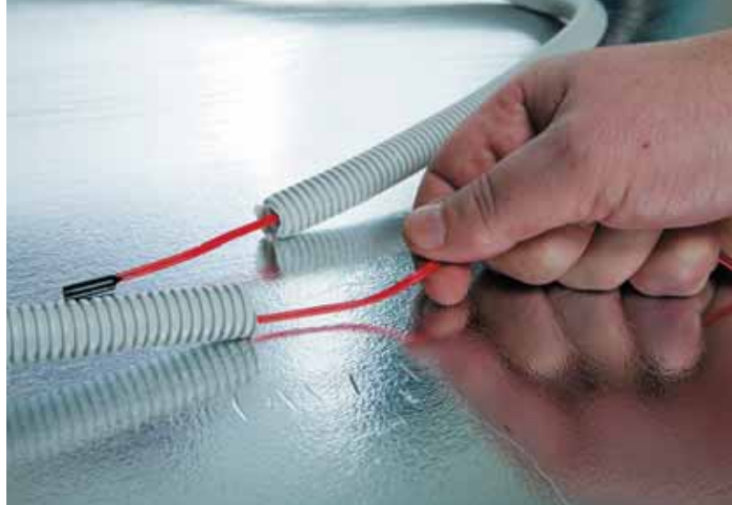
Рис. 16. Установка датчика температуры пола SF-4x15 в гофрированную трубку (конец).
