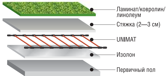
Рис. 21. Схема монтажа теплого пола UNIMAT под ламинат/ковролин/линолеум
