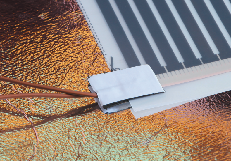
Рис. 20. Вид заизолированного контактного зажима с подключенными проводами
