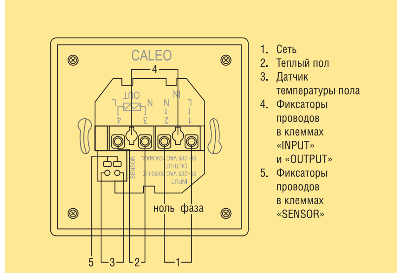
Рис. 21. Пример подключения соединительных проводов к терморегулятору CALEO UTH-10E
