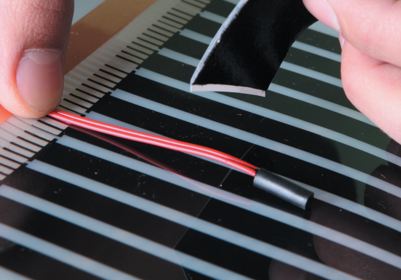
Рис. 24. Датчик прикрепляется к термоплёнке битумной изоляцией
