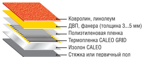
Рис. 4. Схема монтажа теплого пола CALEO под ламинат, ковровин, линолеум
