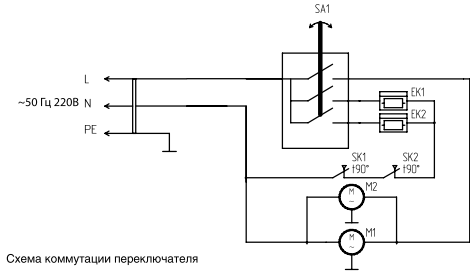
Схема коммутации переключателя
