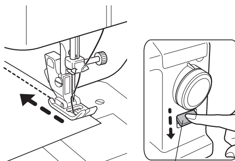
Рычаг реверса
