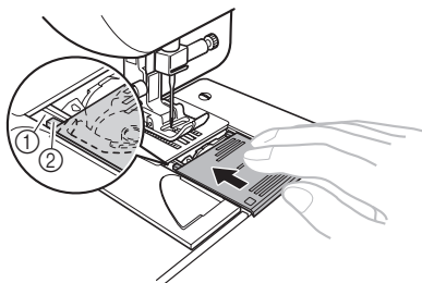
① Вырез ② Выступ
