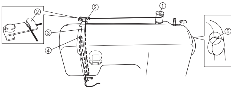
① Стержень для катушки ② Нитенаправитель (сзади) ③ Нитенаправитель (спереди) ④ Рычаг нитепритягивателя ⑤ Метка на маховике
