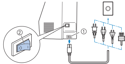
① Гнездо подключения питания ② Кнопка питания
