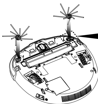
Гнездо и вал боковой щетки
