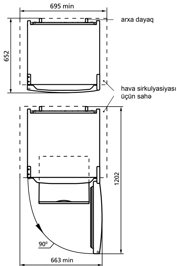
Rəsim 2 – Soyuducu (üstədən görünüşü)
