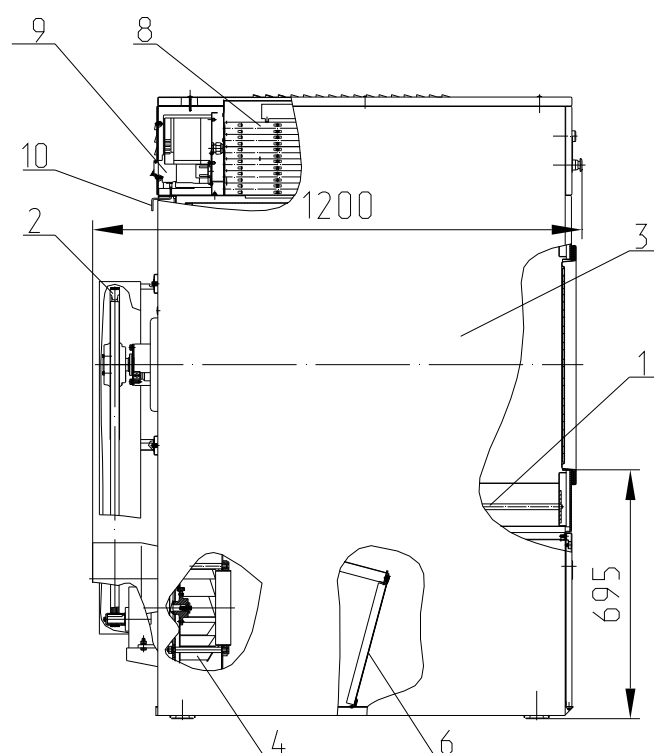
Рис.1. Общий вид
