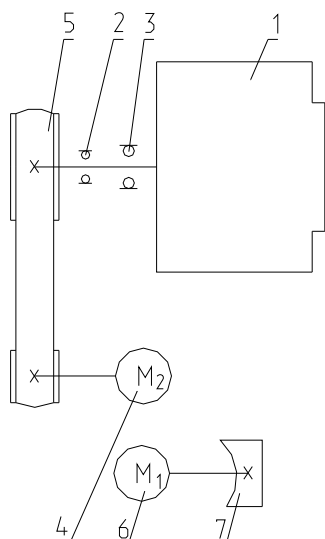
Рис.2. Схема кинематическая
