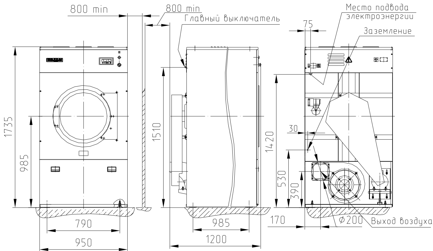
Рис. 5. Монтажный чертеж
