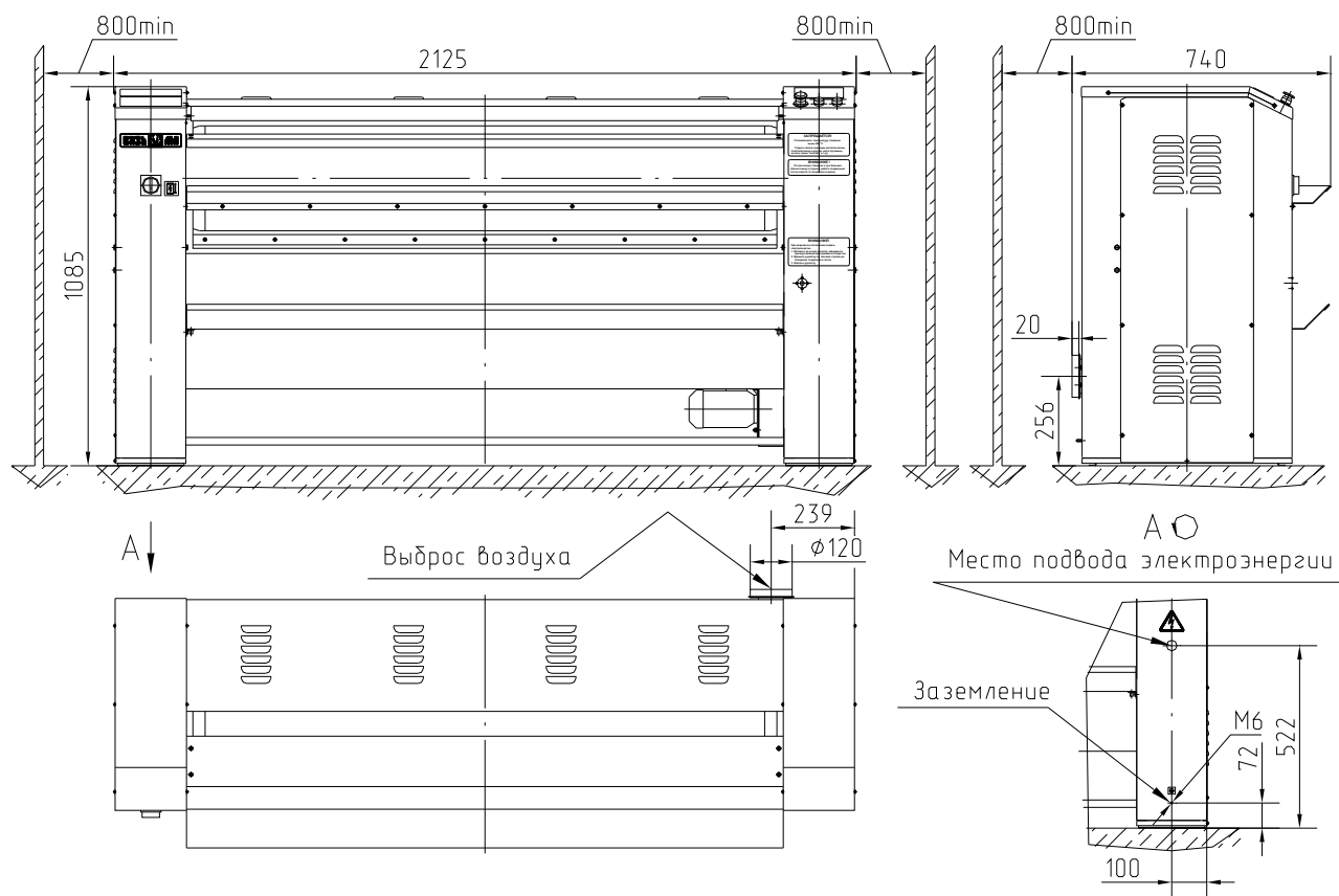
Рис. 7. Монтажный чертеж
