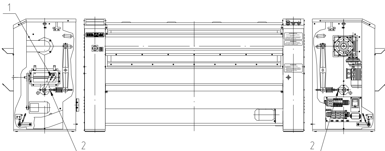
Рис. 8. Схема смазки
