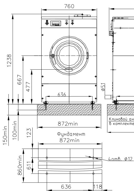
Рис.6 Монтажный чертеж
