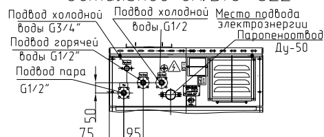
Рис.6 Монтажный чертеж
