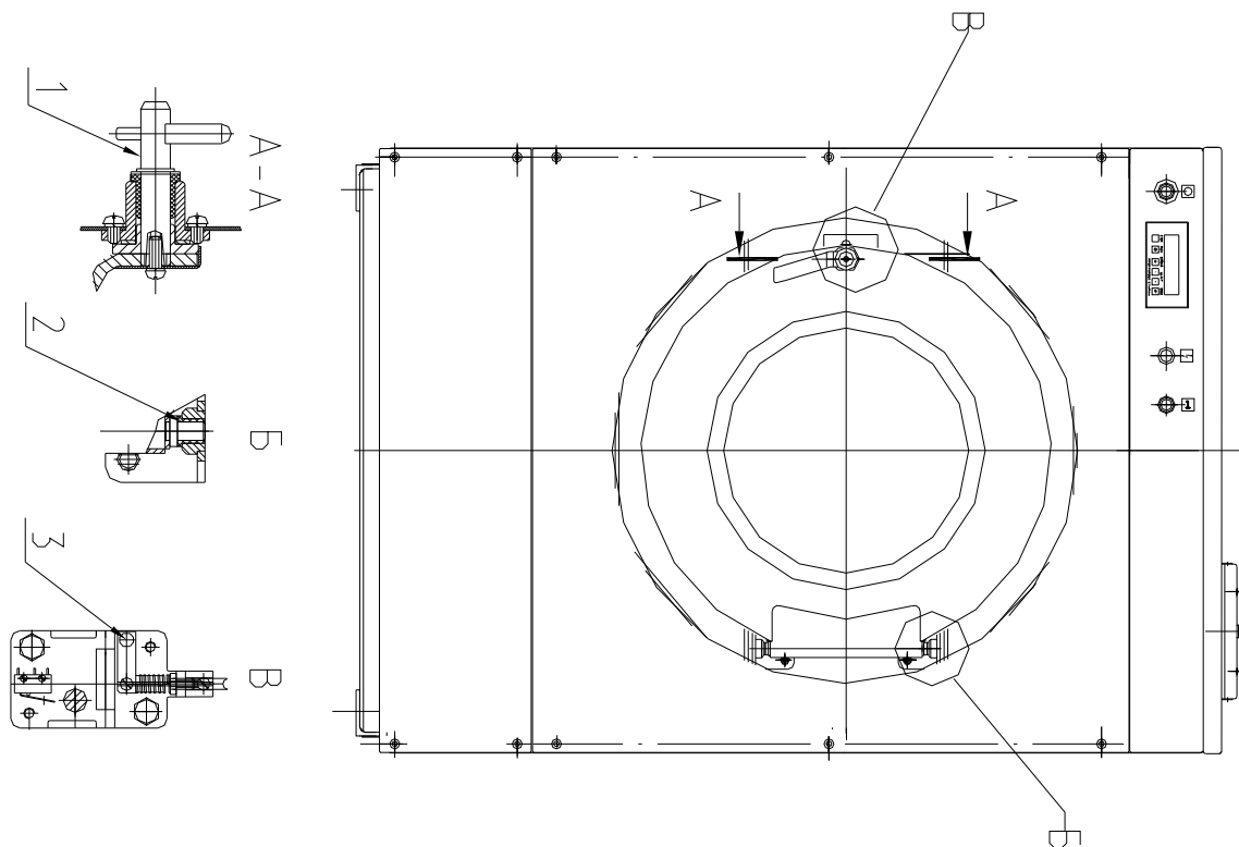
Рис.7 Схема смазки
