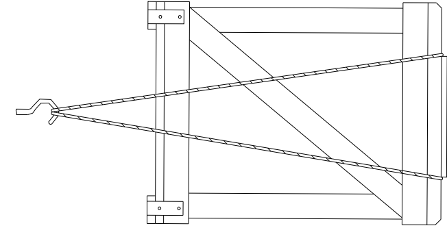
Рис.5 Схема транспортировки
