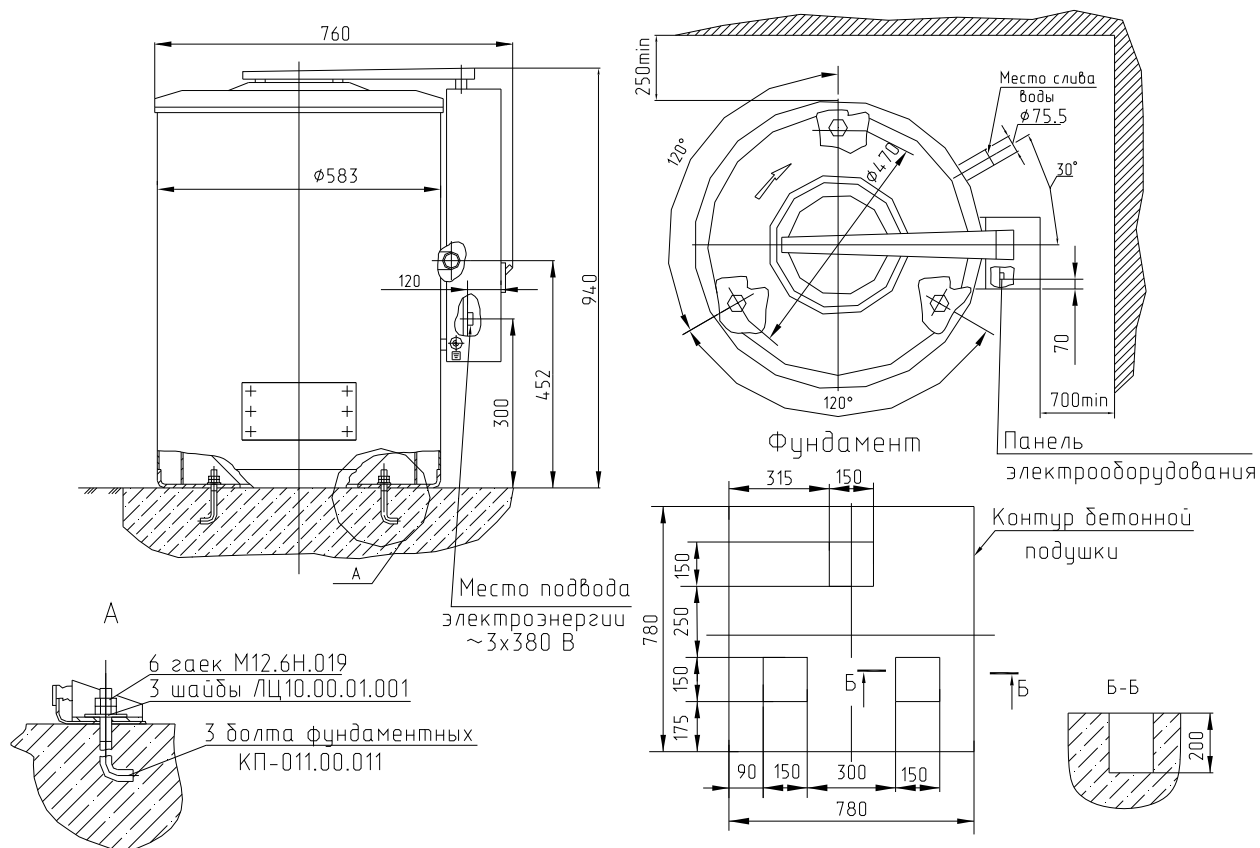
Рис.4 Монтажный чертеж
