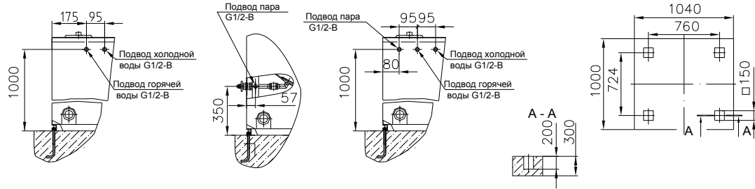
Рис.5 Монтажный чертеж
