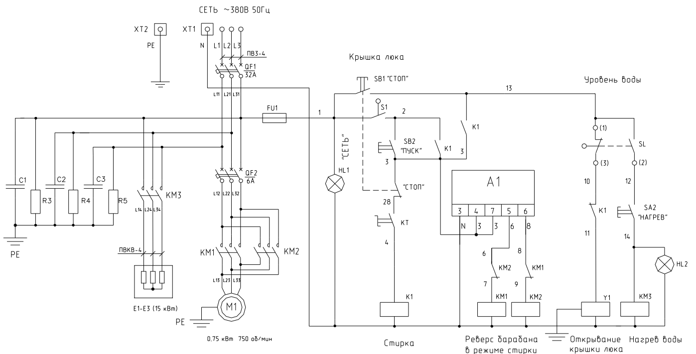
Рис.3в.Схема электрическая принципиальная машины стиральной Л12-121
