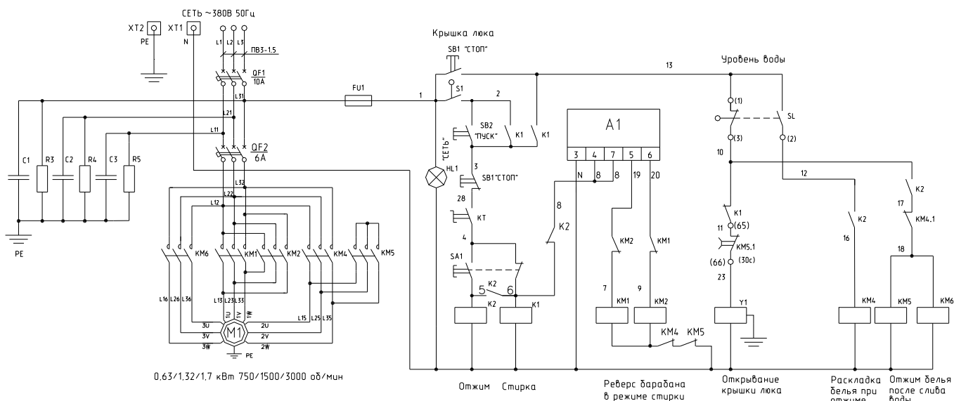
Рис. 3б. Схема электрическая принципиальная машины стиральной Л12-211
