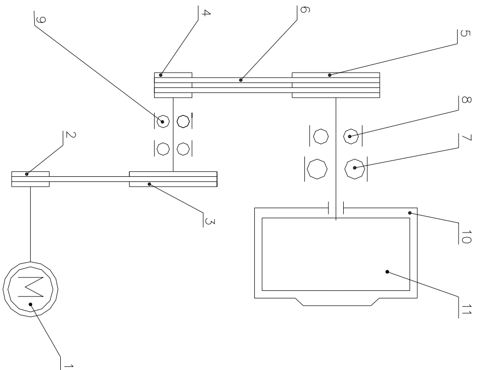
Рис.2 Схема кинематическая
