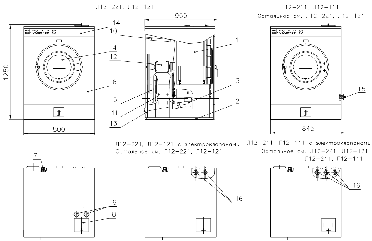
Рис.1 Общий вид
