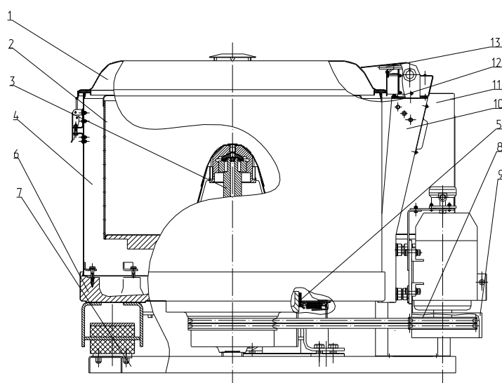
Рис.1 Общий вид
