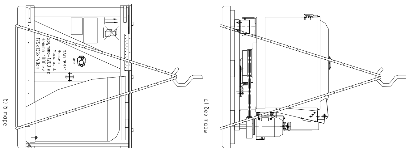
Рис.7 Схема транспортировки
