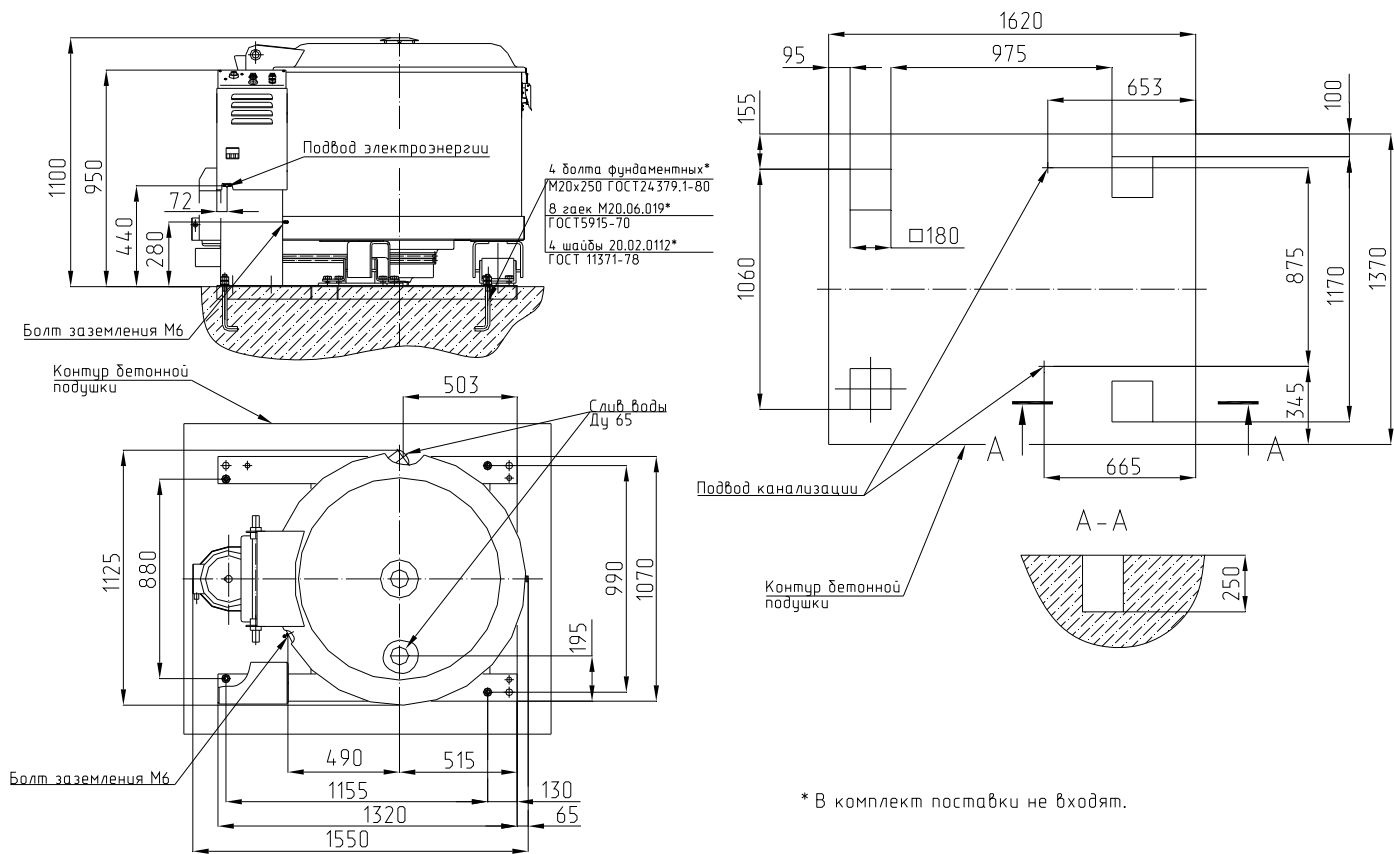
Рис.4 Монтажный чертеж
