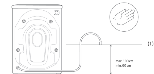
Левосторонний патрубкок
