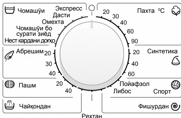
Расми 2 — Дастаи интиҳоби нақшаи шустушӯӣ
