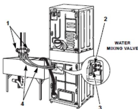
Смесительный клапан
