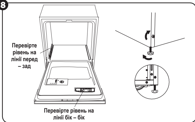
Ілюстрація установаження ніжок.
