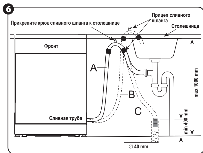
Присоединение сливного шланга. Установите сливной шланг в положении A, B или C.
