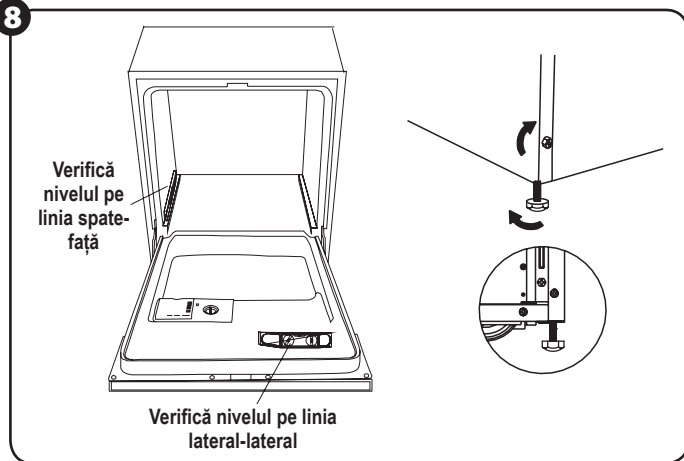
Ilustrația poziționării picioarelor.
