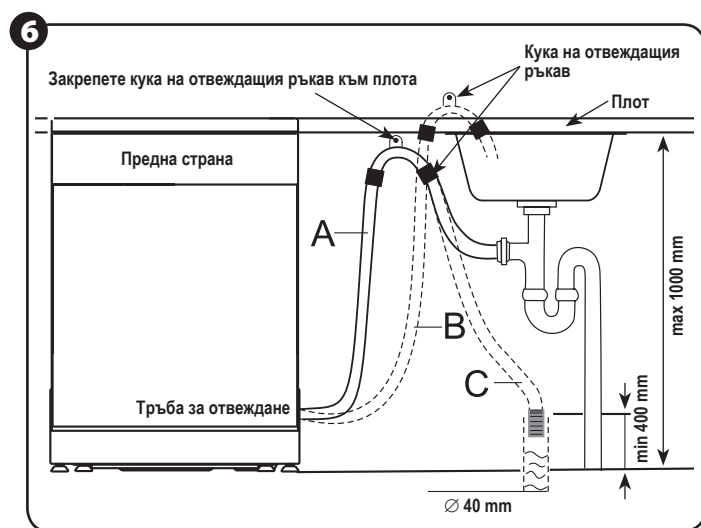
Подключване на отвеждащия ръкав. Монтирайте отвеждащия ръкав в положение A, B или C.
