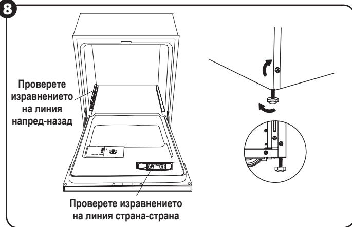
Илюстрация за поставяне на краката.
