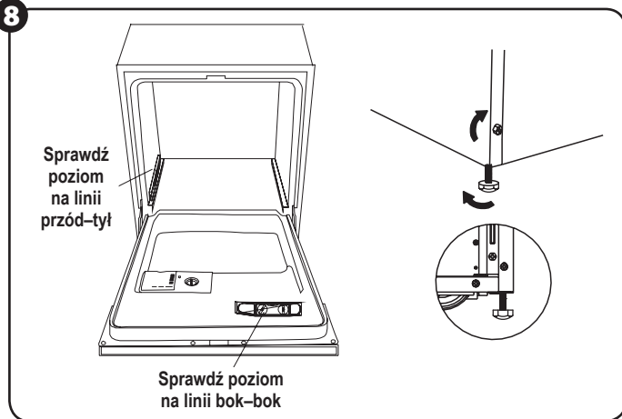
Ilustracja ustawienia nóg.
