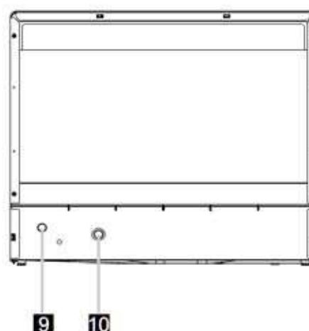
Вид сзади
