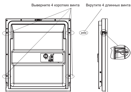
Рис. 4b. Крепление декоративной деревянной панели.
