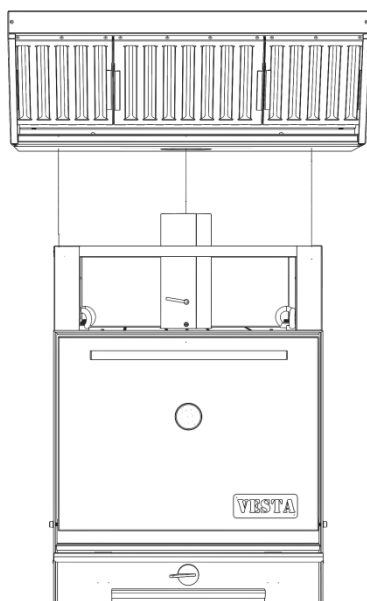
Установка искрогасителя
