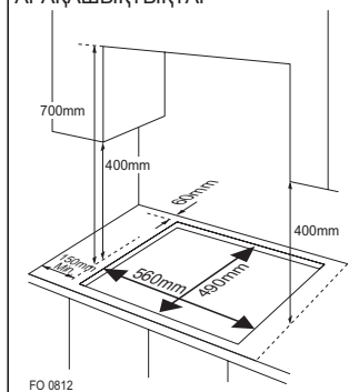
СОҒЫШЫ ЖОҚ ПІСІРУ ПАНЕЛІН ОРНАЛАСТЫРУҒА ҚАЖЕТТІ АРАҚАШЫҚТЫҚТАР
