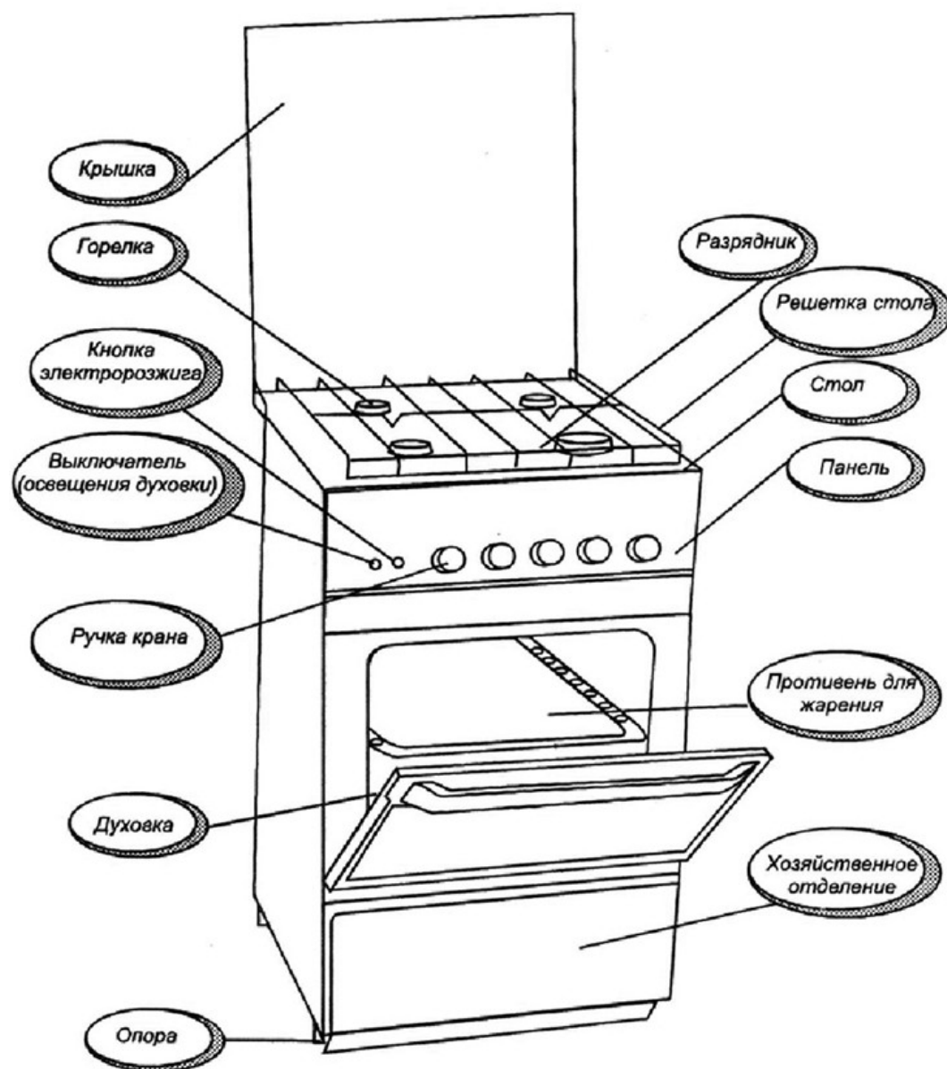
Рис. 1. Устройство плиты
