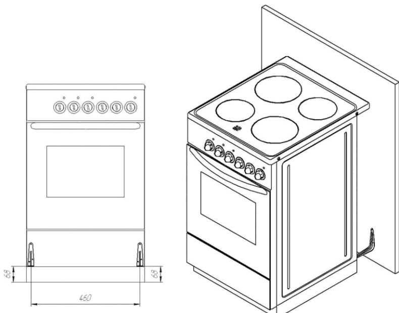
Рис. 5. Схема разметки стены под крошштейны.
