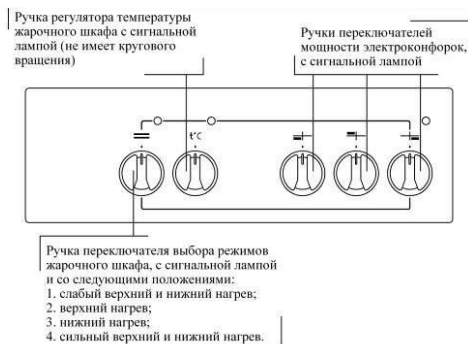
Рис. 7. Передняя панель плиты СТЕ-53 Wh
