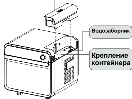
Декоративная панель (водосборник)
