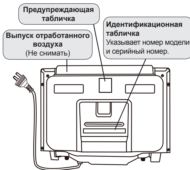
Вид сзади
