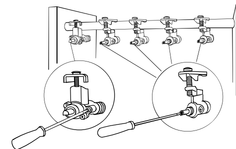
Рисунок А.9 - Регулювання величини малого полум'я/ Рисунок А.9 - Регулирование величины малого пламени/ Şəkil A.9 - Kiçik alov miqdarının tənzimlənməsi/ ნახზო A.9 - მცირე ალის სიდიდის რეგულირება/ A.9-супет - Шағын жалын шамасын реттеу/ Figura A.9 – Reglarea dimensiunii flăcării mici/ A.9-rasm : Kichik alanga hajmini rostlash
