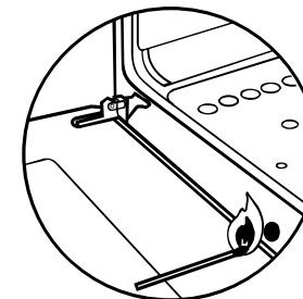
Рисунок А.7 - Ввімкнення пальника духовки/ Рисунок А.7 - Включение горелки духовки/ Şəkil A.7 - Soba odluğunun yandırılması/ ნახზო A.7 - ღუმელის საწებურას ჩართვა/ A.7-супет - Духовканың жанарғысын қосу/ Figura A.7 – Pornirea arzătorului cuptorului/ A.7-rasm : Dухovkaniy yondirgichi (gorelka)ni yoqish
