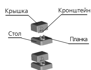
Рисунок 4 - Схема крепления металлической крышки
