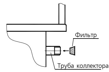
Рисунок 6 - Схема установки фильтра (для газовых плит, оснащенных автоматом безопасности)
