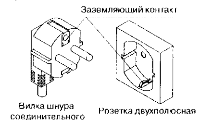
Рисунок 1 — Заземление плиты
