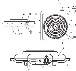
Рисунок 1 — Модель 111Т
