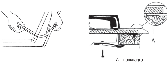
A – прокладка
