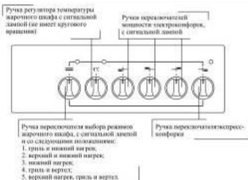
Рис. 11. Передняя панель плиты ЭП4/1э03
