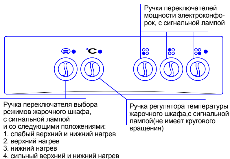
Рис. 4 Передняя панель плиты ЭП301МС
