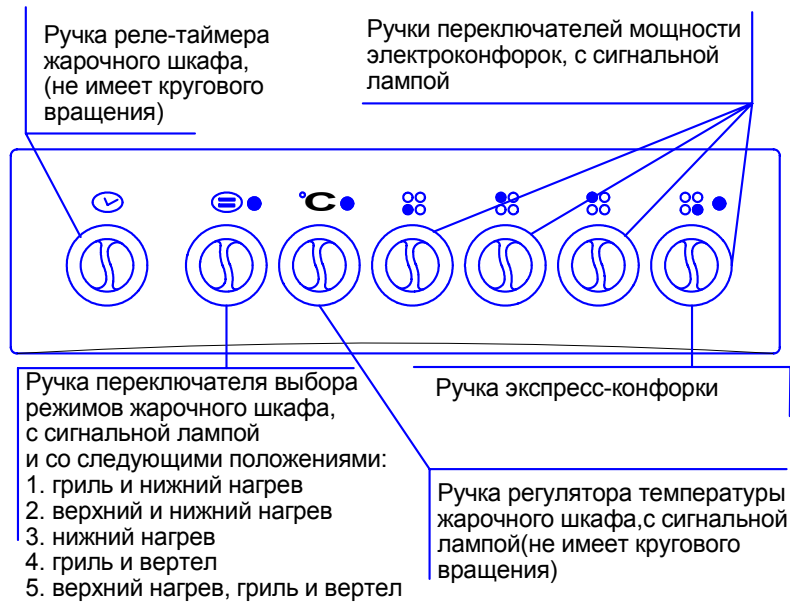
Рис. 10 Передняя панель плиты ЭП4/1333МС
