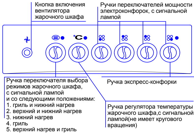
Рис. 9 Передняя панель плиты ЭП4/1304МС
