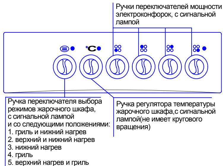
Рис. 5 Передняя панель плиты ЭП402МС
