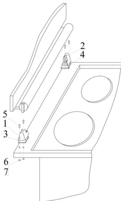
Рис. 2 Установка стеклянной крышки стола.
