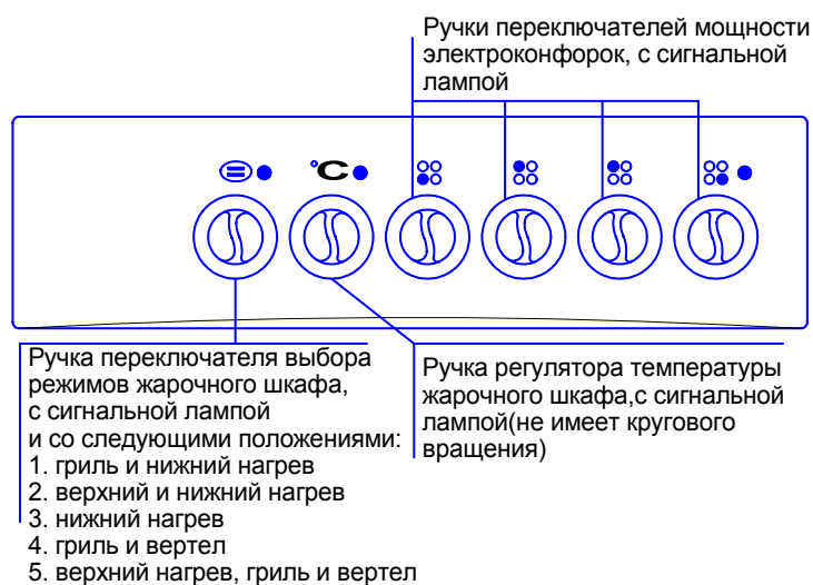
Рис. 6 Передняя панель плиты ЭП403МС
