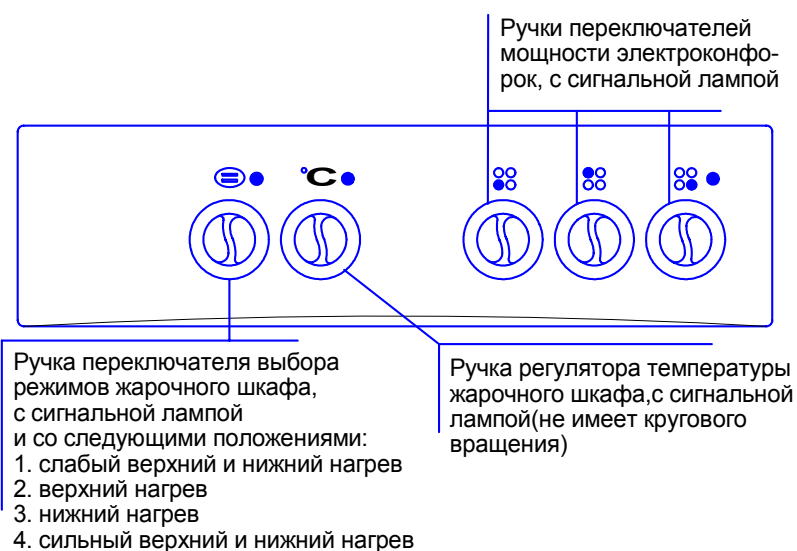
Рис. 4 Передняя панель плиты ЭП301МС
