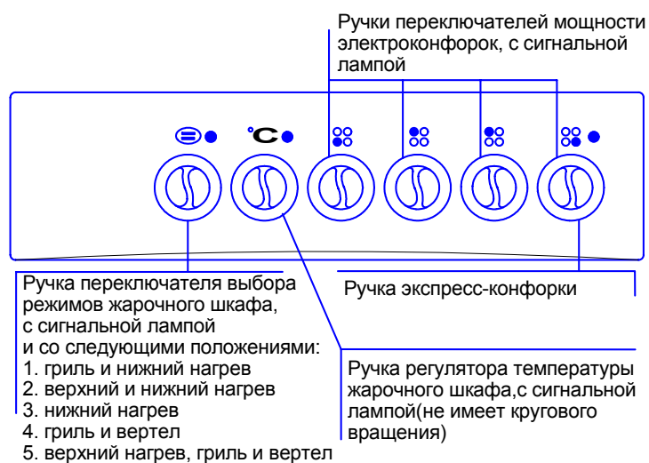
Рис. 8 Передняя панель плиты ЭП4/1Э03МС
