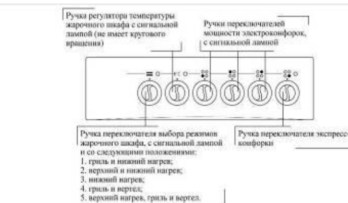
Рис. 12. Передняя панель плиты ЭП4/1э03МС, ЭП4/1э03М2С
