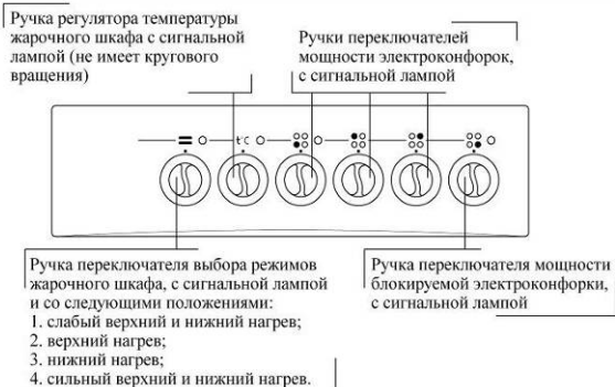
Рис. 11. Передняя панель плиты ЭП411МС, ЭП411М2С
