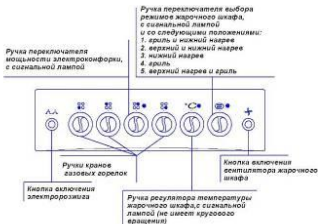
Рис. 14. Передняя панель плит ЭГ1/3г14МС-2у; ЭГ1/3г14М2С-2у
