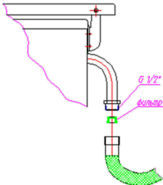
Подсоединение с помощью гибкого присоединительного рукава
