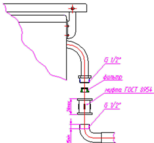
Жесткое подсоединение плиты к газовому стояку
