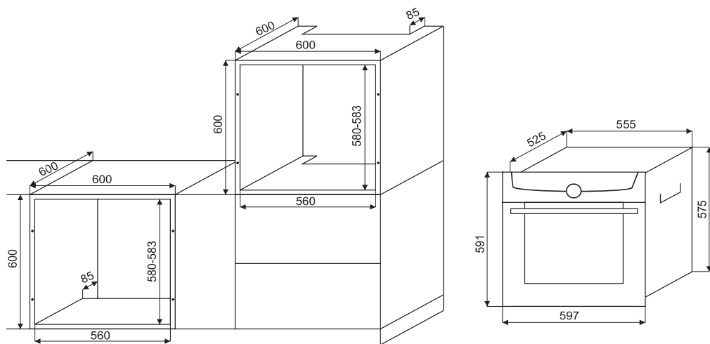
Рис. 6. Схема по встраиванию духового шкафа
