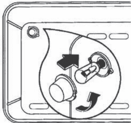
Рис. 9. Замена лампы
