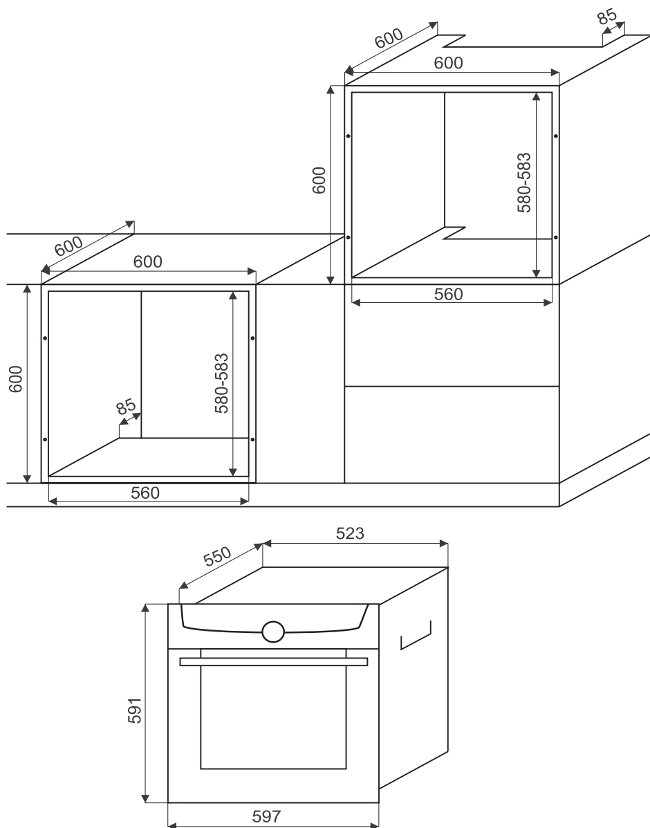
Рис. 7. Схема по встраиванию духового шкафа
