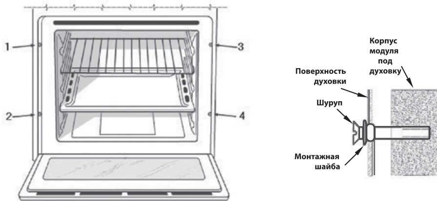
Рис. 8. Крепление духового шкафа к мебели
