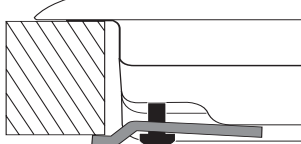
Posizione gancio per top H=40mm
