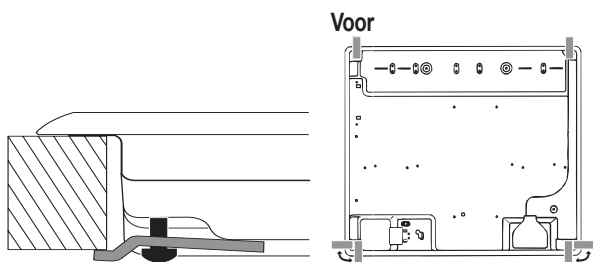
Stand haak voor keukenblad H=40mm
