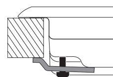
Монтаж крюка для опорных брусьев Н=30мм
