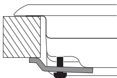
تركيب الخطافات بالنسبة للسطح الارتفاع=30 ملم
