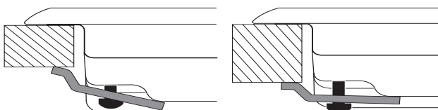
Posição do gancho para H=20mm
