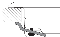
تركيب الخطافات بالنسبة للسطح الارتفاع=20 ملم
