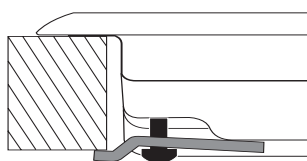
Posición del gancho para superficies H=40\text{mm}
