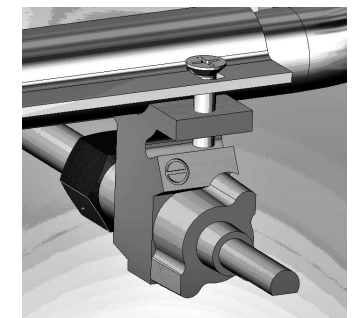
Мал. 6 Кран газовий з гвинтом малого полум'я
