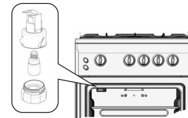
Мал. 13 Заміна лампи освітлення
