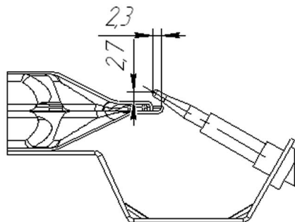
Рис. 14 Расположение термопары горелки духовки.
