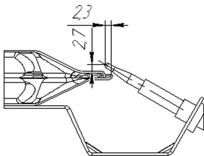
Мал. 14 Розташування термopapи пальника духовки.
