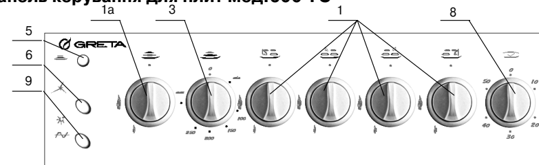
Мал. 8 Панель керування
