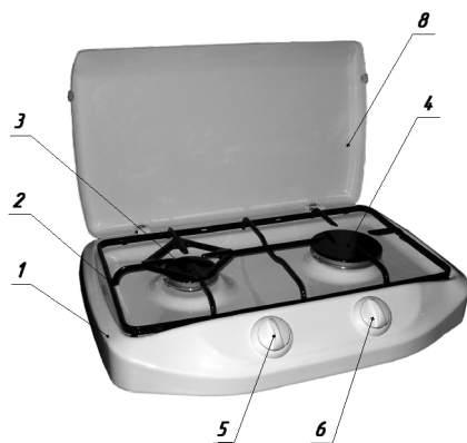
Рис. 1 Устройство плиты
